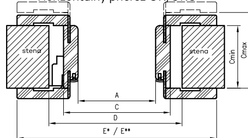
Horizontálny prierez OR/ORC
